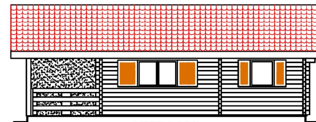
ELEWACJA 3-2
