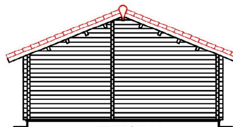
ELEWACJA 2-1
