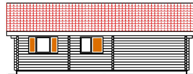
ELEWACJA 1-4
