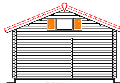
ELEWACJA 1-2
