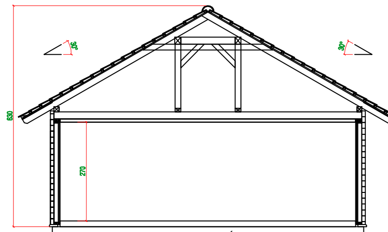
PRZEKRÓJ
