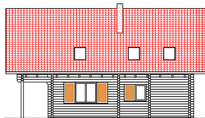
ELEWACJA 1-4
