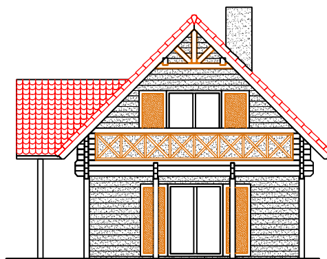
ELEWACJA 2-1
