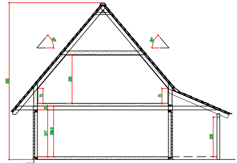
PRZEKRÓJ
