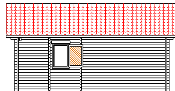
ELEWACJA 2-1
