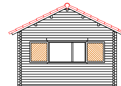
ELEWACJA 1-4
