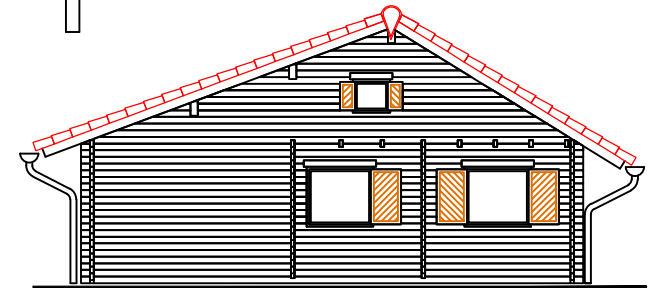
ELEWACJA 4-3
