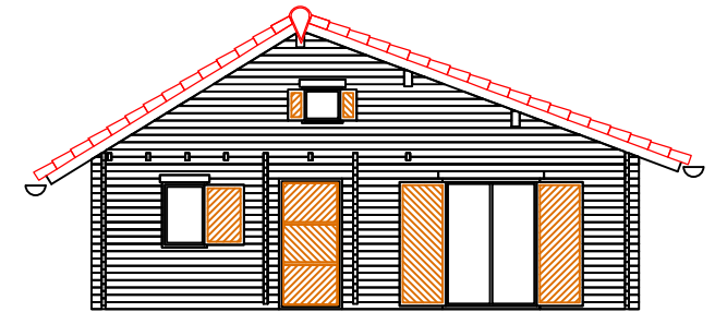
ELEWACJA 2-1
