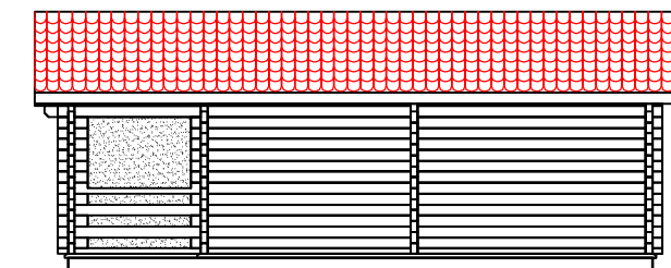
ELEWACJA 4-3
