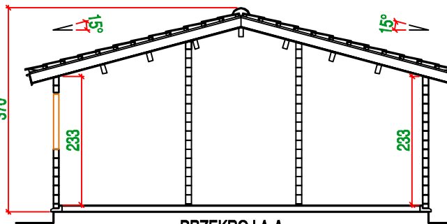
PRZEKROJ A-A
