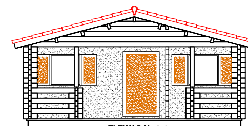
ELEWACJA 1-4
