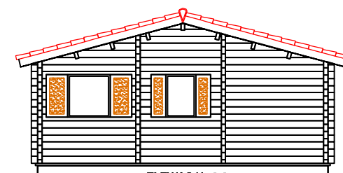
ELEWACJA 3-2
