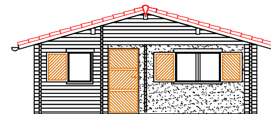
ELEWACJA 1-4
