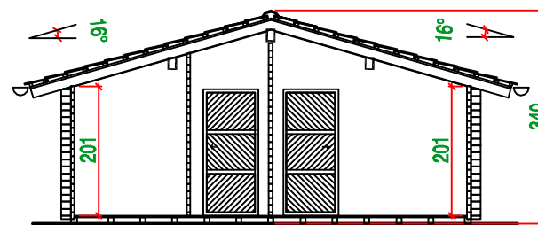
PRZEKRÓJ A-A
