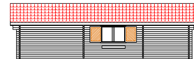
ELEWACJA 2-1
