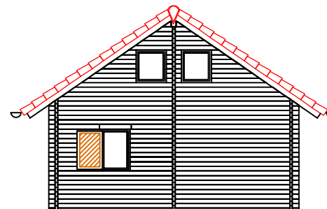
ELEWACJA 2-3
