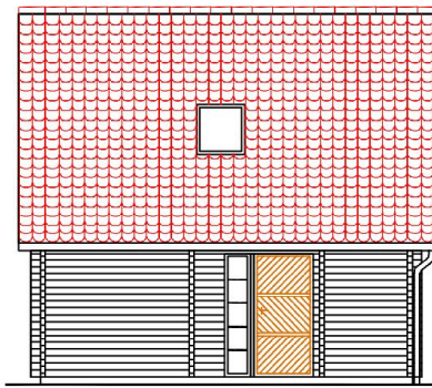
ELEWACJA 2-3
