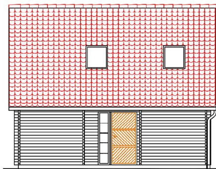
ELEWACJA 3-2
