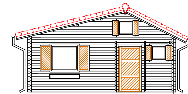
ELEWACJA 1-2
