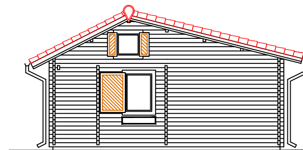
ELEWACJA 3-4
