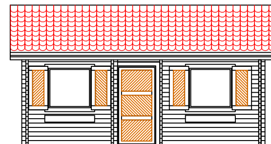
ELEWACJA 1-2
